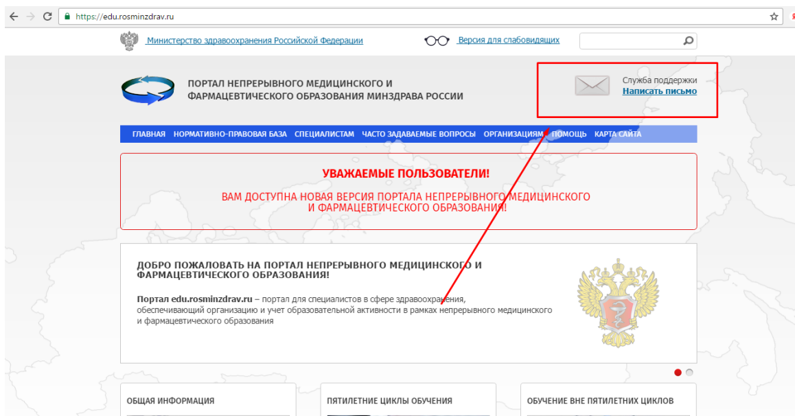
Рисунок 9 – «Служба поддержки»
